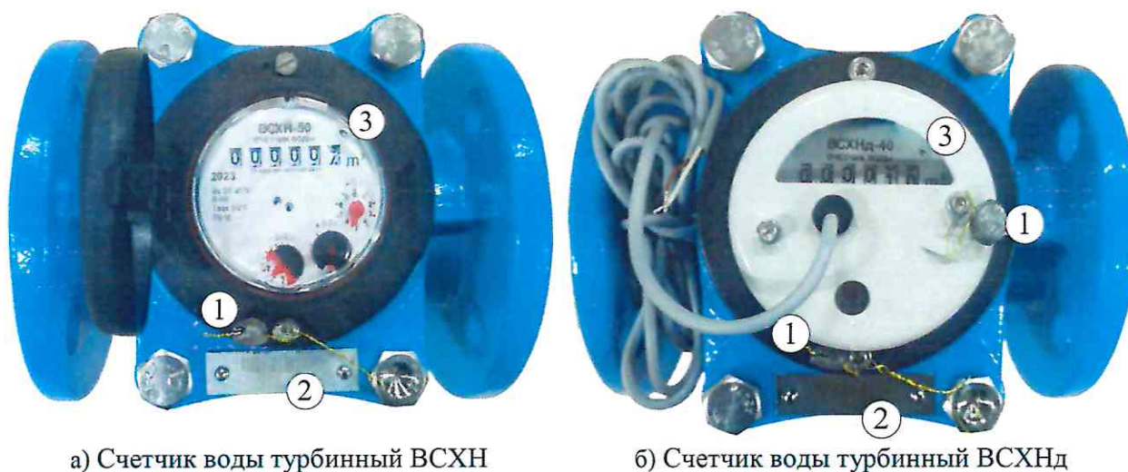
Рисунок 2 – Схема пломбировки от несанкционированного доступа и места нанесения заводского номера и знака утверждения типа
