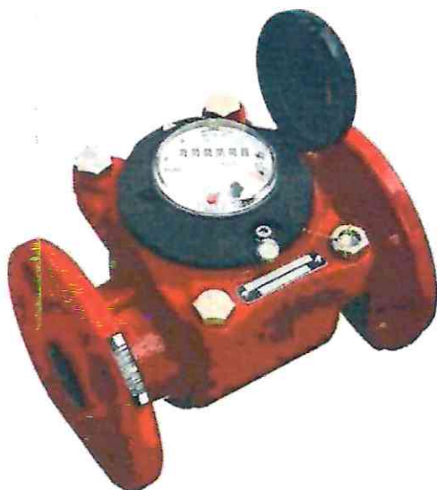
в) Счетчик воды турбинный ВСГН, на примере ВСГН-50
