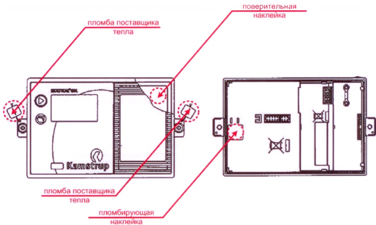
Рисунок 2 - Схема пломбировки теплового счетчика MULTICAL® 602 и место нанесения отметки о проверке
